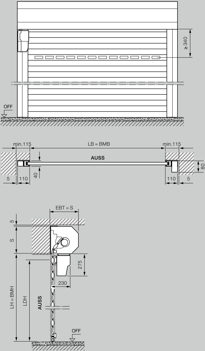
Zakres wymiarów bramy rolowanej wewnątrz i na zewnątrz
