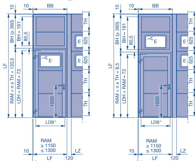
Przeszklenie sandwich typ E TH = 625
