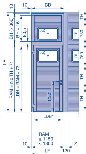
Przeszklenie sandwich typ E TH = 750
