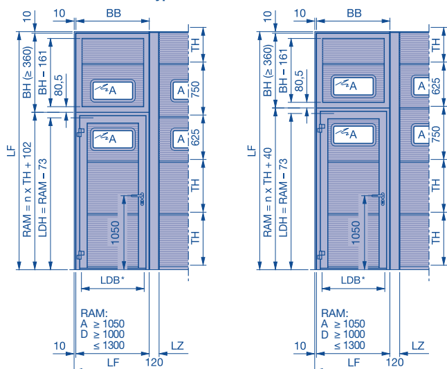
Przeszklenie sandwich typ E TH = 750
