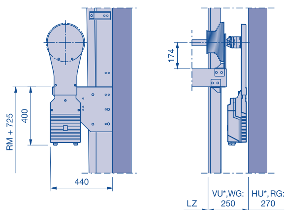
Przykład montażowy ⑧ z prawej strony
