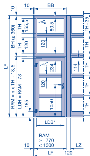
Drzwi boczne NT 60 takie same jak bramy typu ALR F42 Thermo
