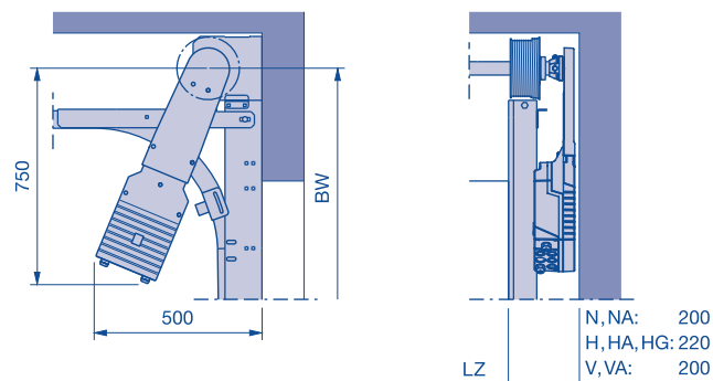
Przykład montażowy ⑨ z prawej strony
