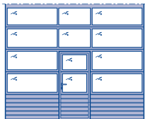
Brama segmentowa APU F42 z drzwiami przejściowymi bez wystającego progu
