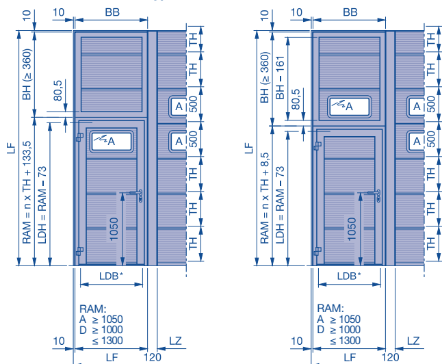
Przeszklenie sandwich typ A TH = 625 / 750 i 750 / 625
