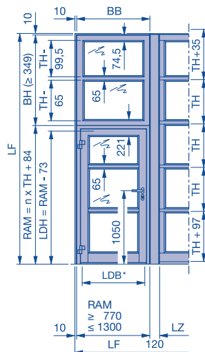
Drzwi boczne NT 60 takie same jak bramy typu ALR F42 S-Line
